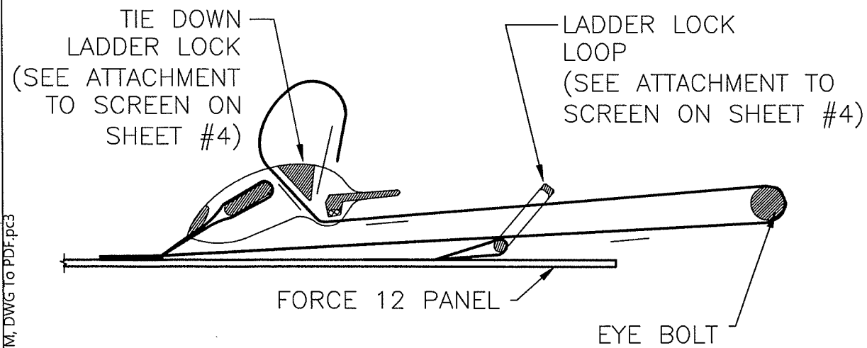
2 STRAP PATH - THROUGH BUCKLE D1 SCALE: N.T.S. = 1'-0"
