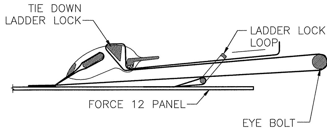
4 STRAP PATH - THROUGH LOOP D1 SCALE: NTS = 1'-0"
